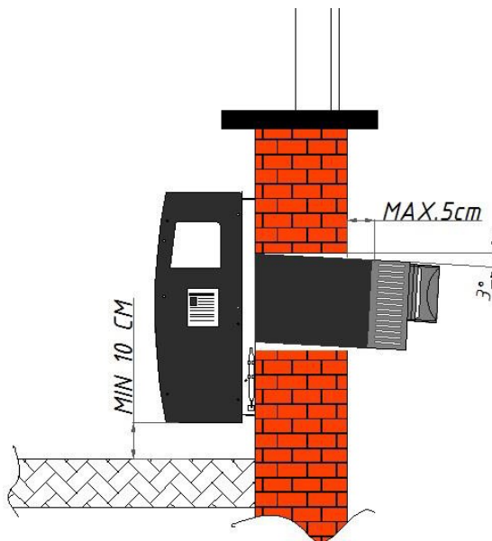
Рисунок-5: Схема монтажа конвектора HP/HS
