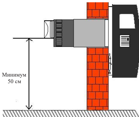
Рисунок 1: Расстояние отверстия дымовой трубы от земли.
