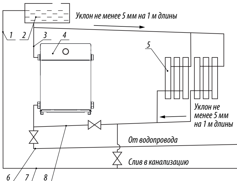
Рисунок 7. Рекомендуемая схема системы отопления без циркуляционного насоса
