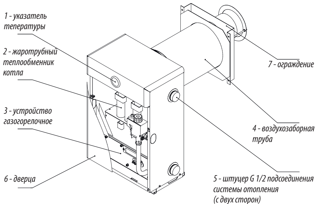
Рисунок 5. Воздухозаборная труба с каналом дымоудаления
