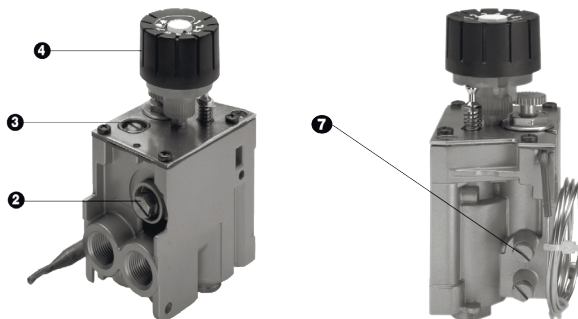
Рисунок 8. Элементы регулировки газового клапана 630 EUROSIT и TGV-307
