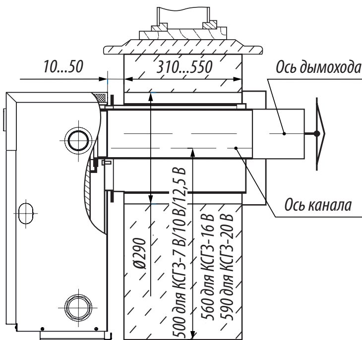
Рисунок 6. Схема установки котла КСГЗ
