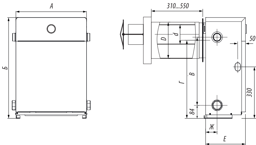
Рисунок 1. Общий вид, габаритные и присоединительные размеры котлов
