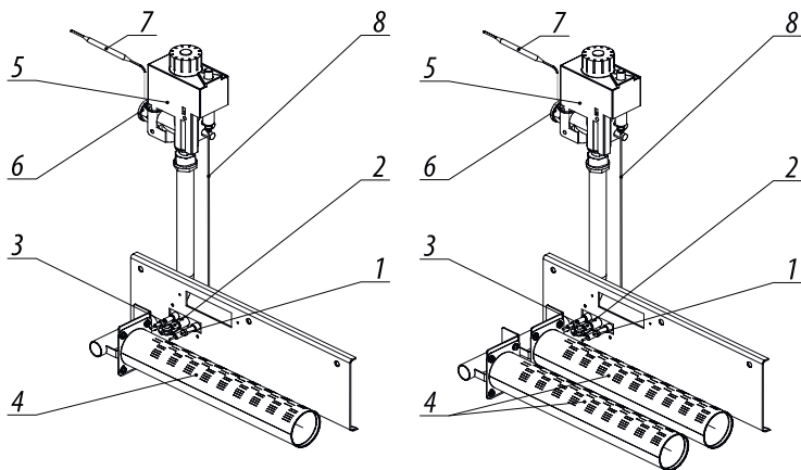
Рисунок 3. Устройство газогорелочное с газовым блоком EUROSIT 630 и TGV-307
